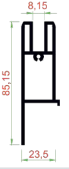
TGT-107 AÇILIR CAM BAZA (TEK CAM) 0.886 KG/M
