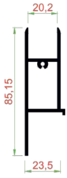
TGI-107 AÇILIR CAM BAZA (ISI CAM) 0.886 KG/M
