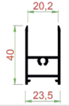
TGI-105 BAZA (ISI CAM) 0.629 KG/M
