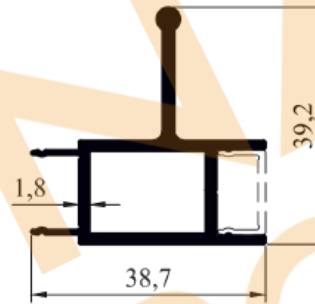
1700-211 KASA 0.610 KG/M
