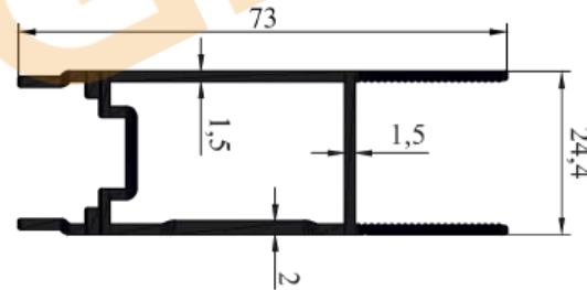
1700-212 BAZA 0.860 KG/M
