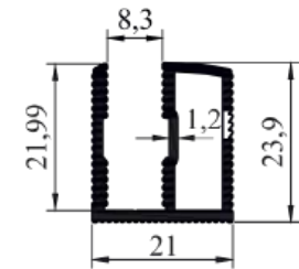
1700-194 BEMUS 8MM U 0.395 KG/M
