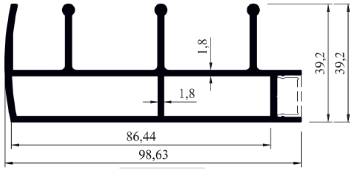
1700-210 KASA 1.705 KG/M
