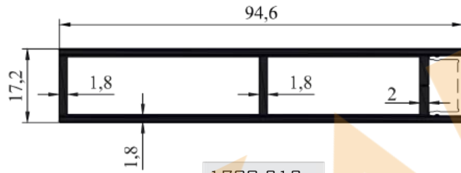
1700-213 YAN KASA 1.135 KG/M
