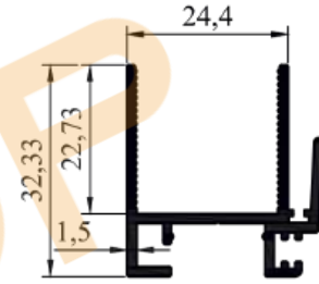
1700-216 SÜRME KENET 0.485 KG/M
