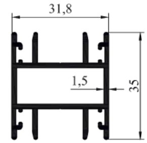
1700-215 SÜRME KENET 0.715 KG/M
